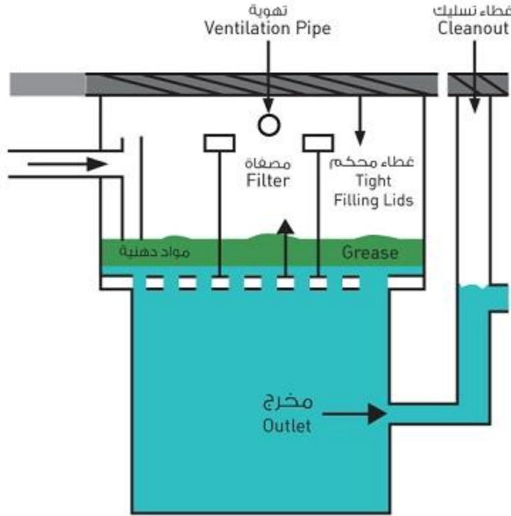
رسم توضيحي لمصيدة الدهون Grease Trap Design
